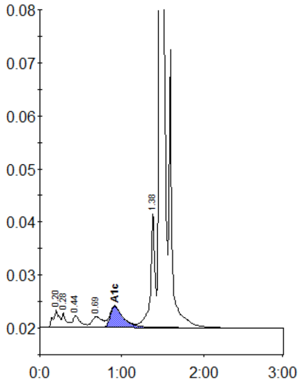
Peak table - ID: 10349601
